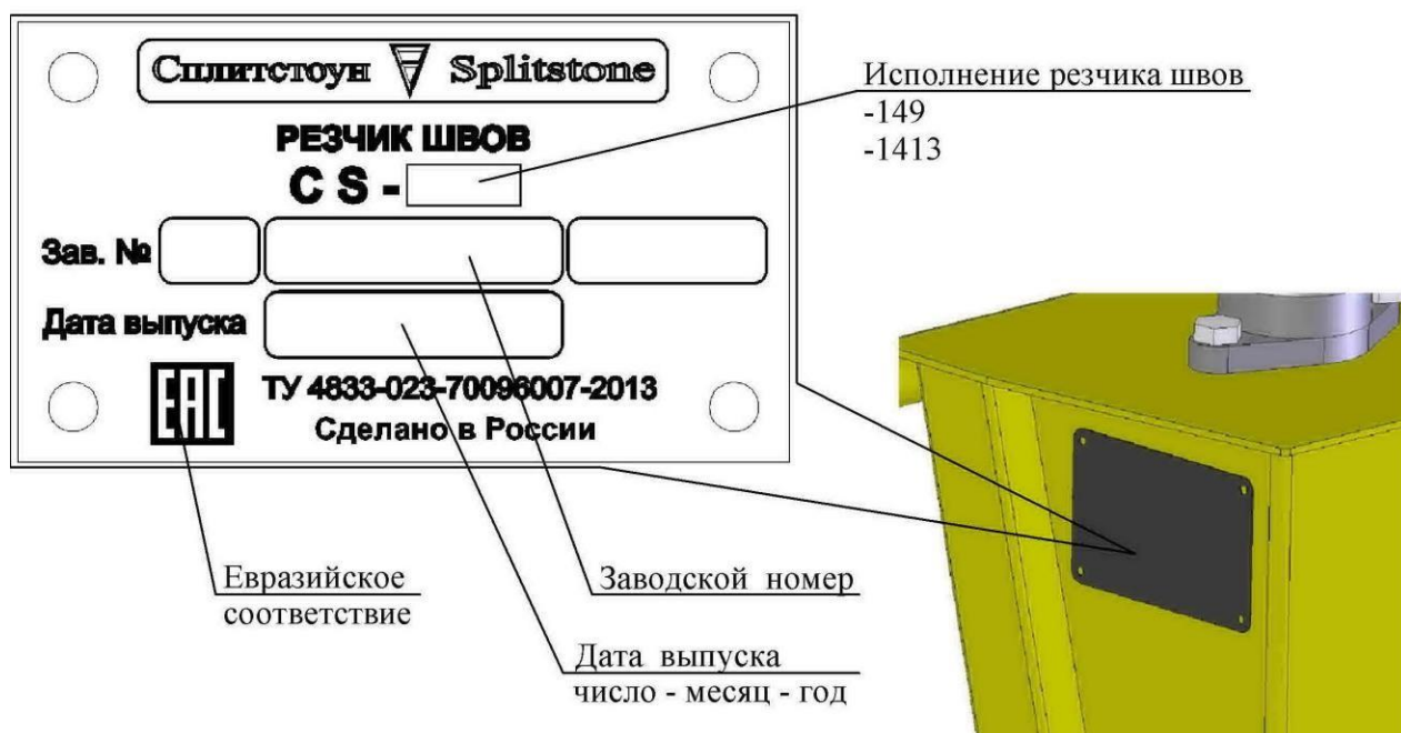
Рисунок 2 - Маркировка
