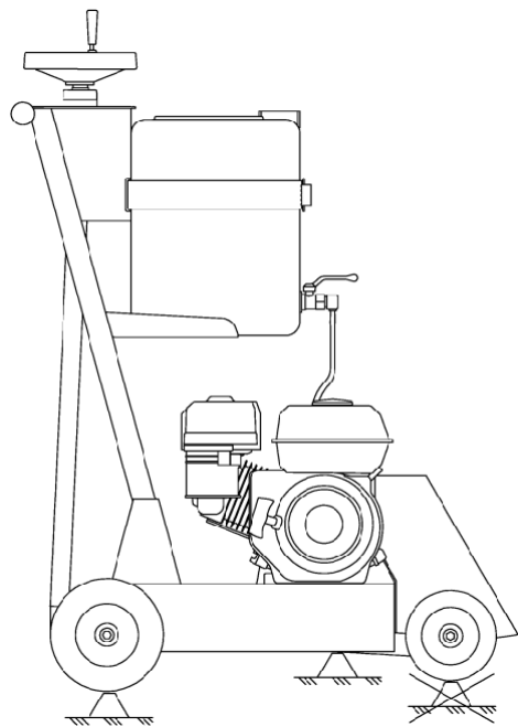
Рисунок 11 – Схема установки резчика при транспортировании
